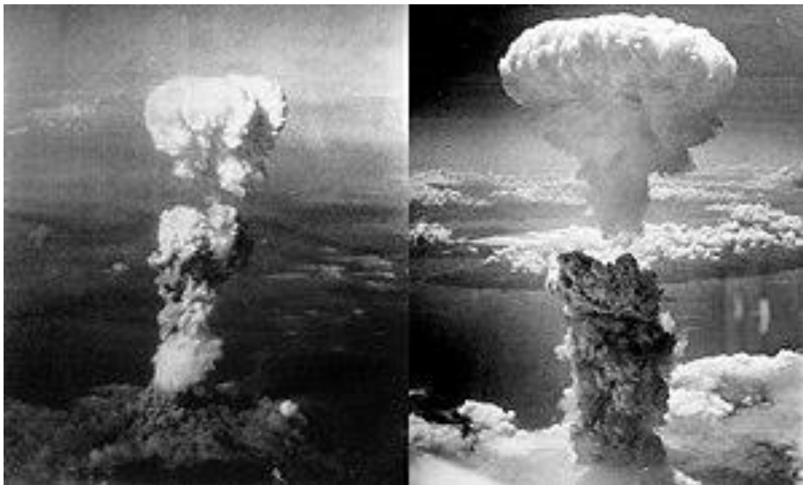
Ядрените взривове над Хирошима и Нагасаки
